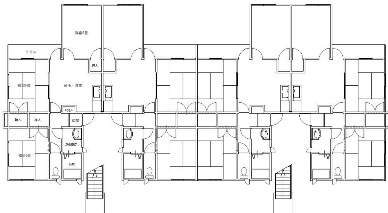
F - 1 棟 平面図
